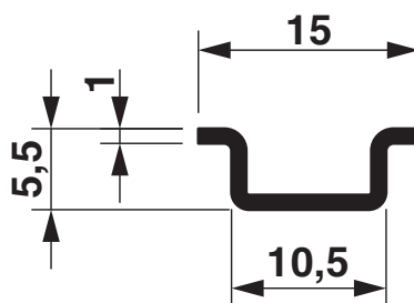
Rysunek wymiarowy
