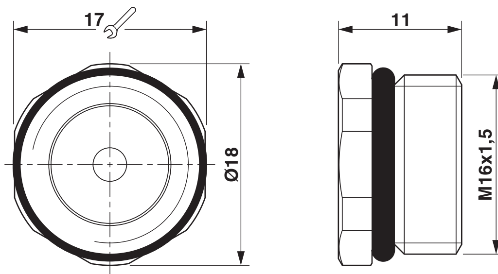
Rysunek wymiarowy
