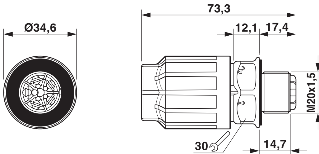
Rysunek wymiarowy QPD W 5x2,5 M20
