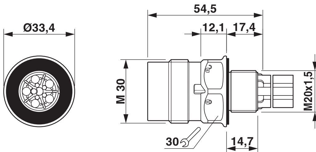
Rysunek wymiarowy QPD W 5x2,5 M20 bez nakrętki
