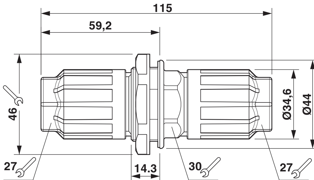
Rysunek wymiarowy QPD CW 5x2,5
