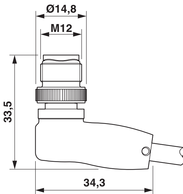
Rysunek wymiarowy
