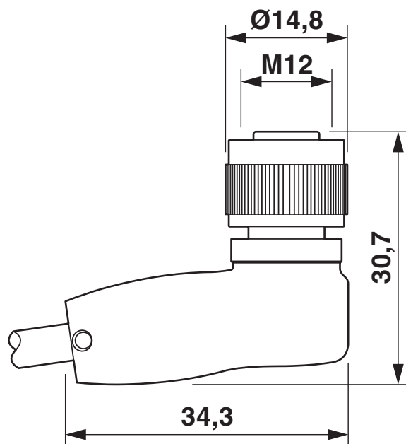
Rysunek wymiarowy
