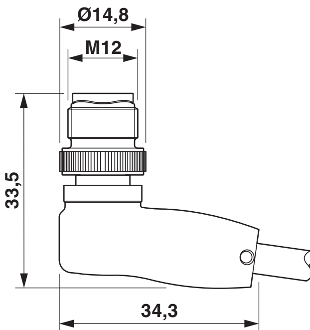
Rysunek wymiarowy
