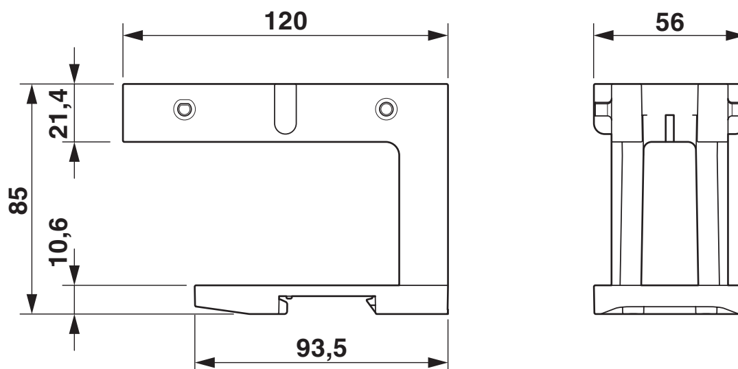
Rysunek wymiarowy
