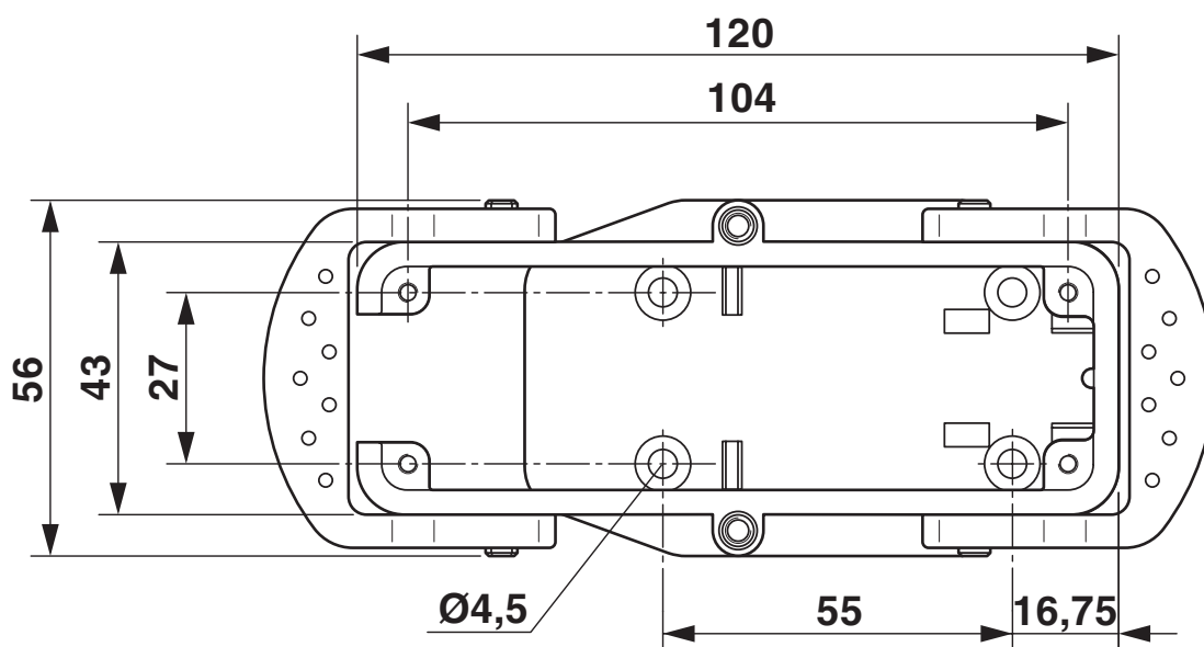
Rysunek uproszczony z ważniejszymi wymiarami (widok z góry)
