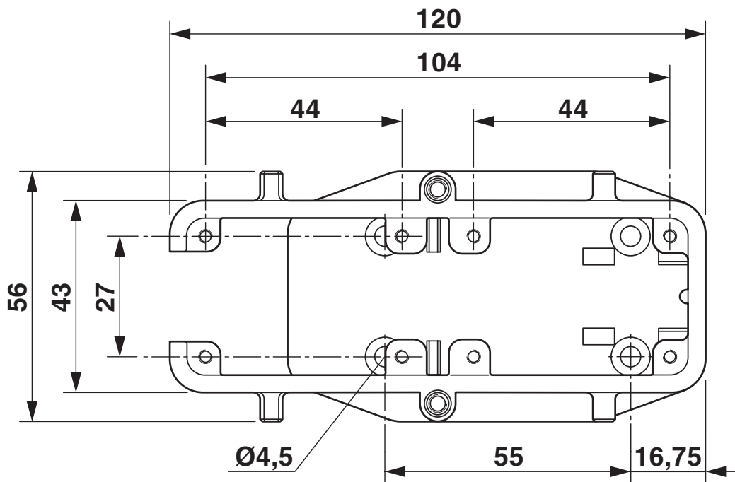
Rysunek uproszczony z ważniejszymi wymiarami (widok z góry)
