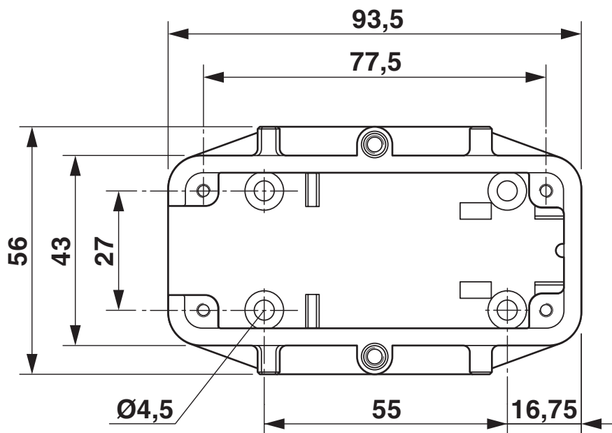
Rysunek uproszczony z ważniejszymi wymiarami (widok z góry)
