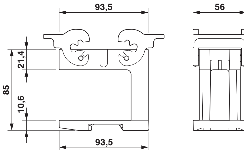
Rysunek wymiarowy
