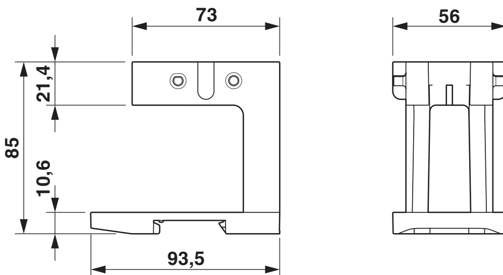
Rysunek wymiarowy
