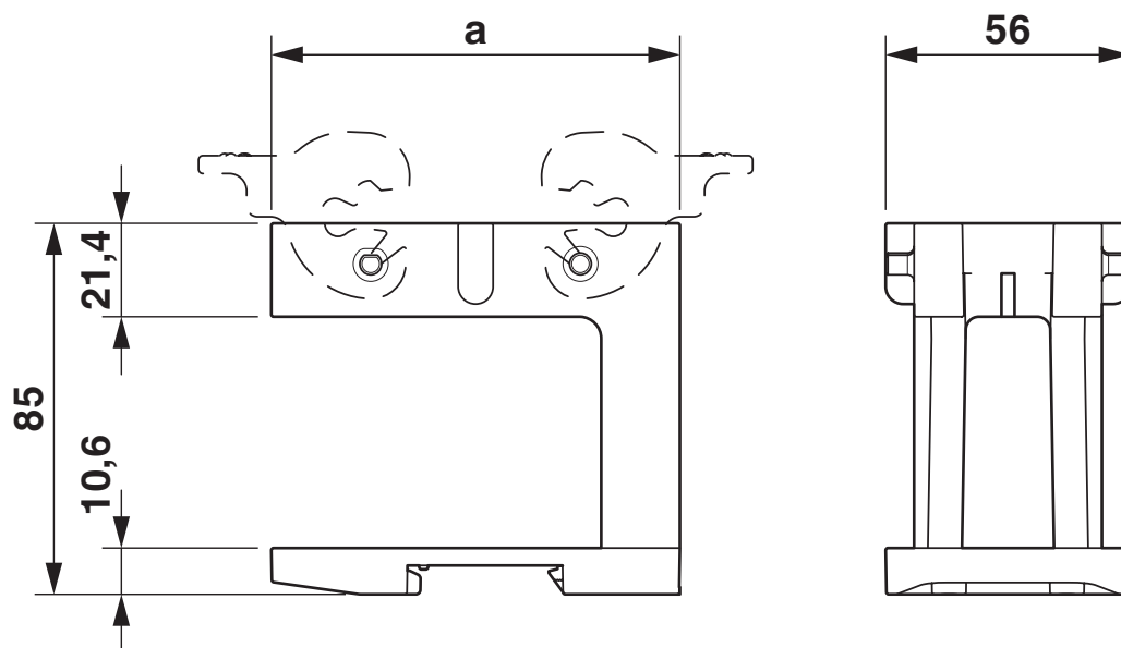
Rysunek wymiarowy
