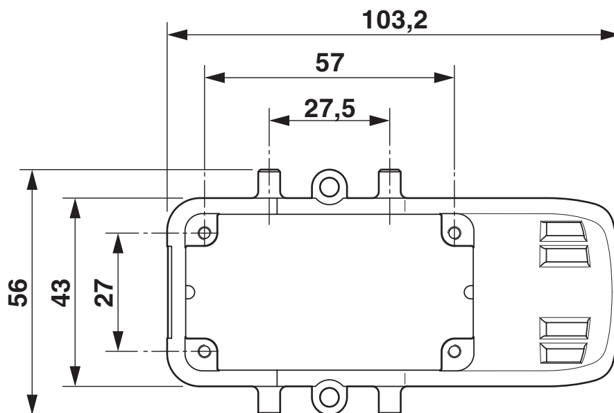
Rysunek wymiarowy
