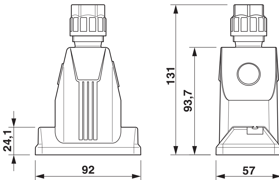
Rysunek wymiarowy
