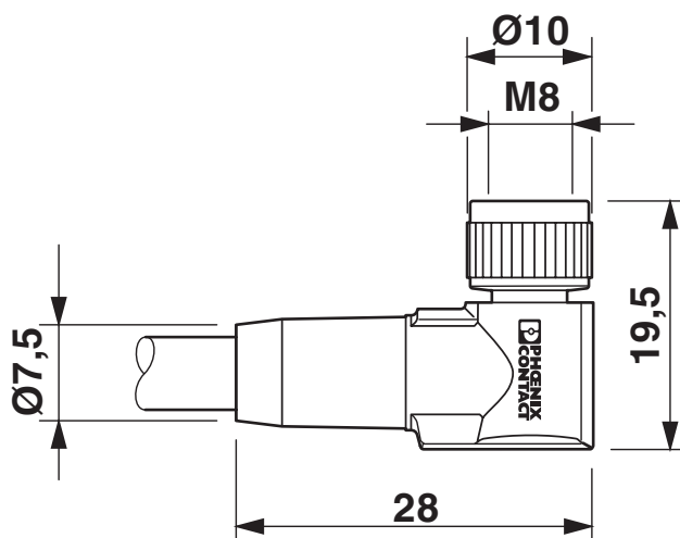
Rysunek wymiarowy
