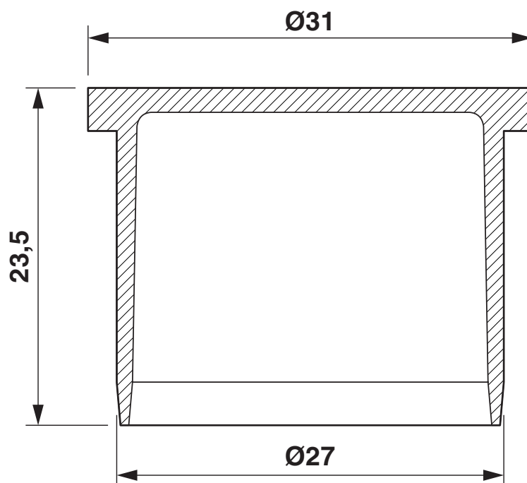
Rysunek wymiarowy
