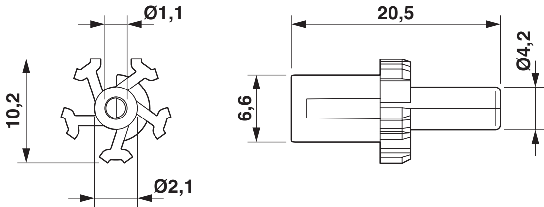
Rysunek wymiarowy
