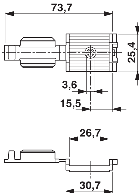
Rysunek wymiarowy
