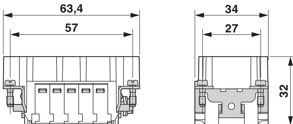
Rysunek wymiarowy
