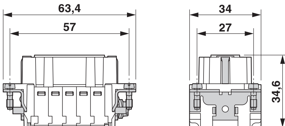
Rysunek wymiarowy
