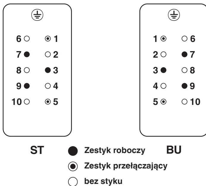
Rysunek schematyczny
