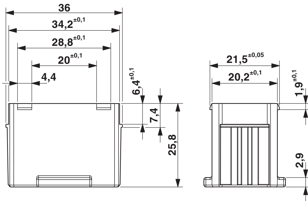
Rysunek wymiarowy
