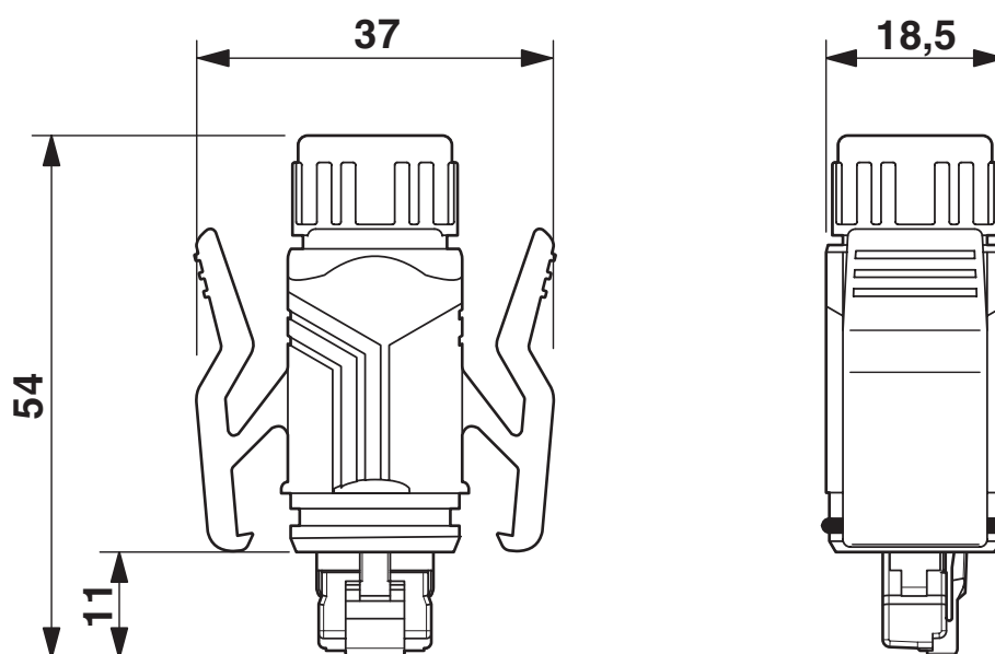
Rysunek wymiarowy
