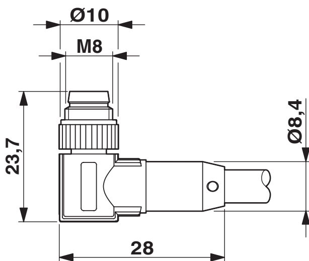
Rysunek wymiarowy
