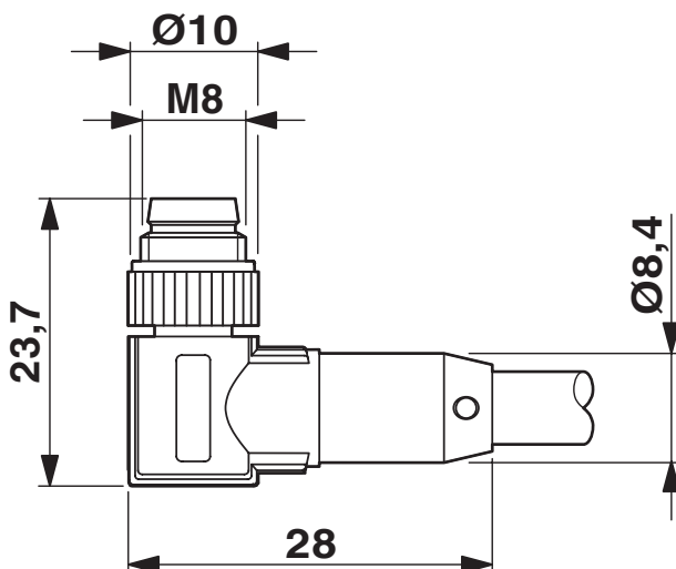
Rysunek wymiarowy
