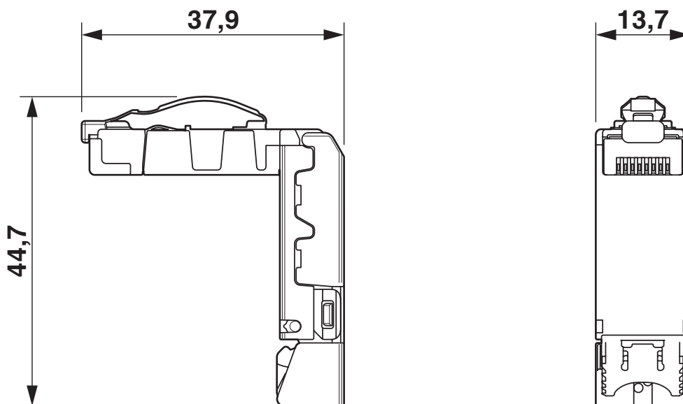
Rysunek wymiarowy
