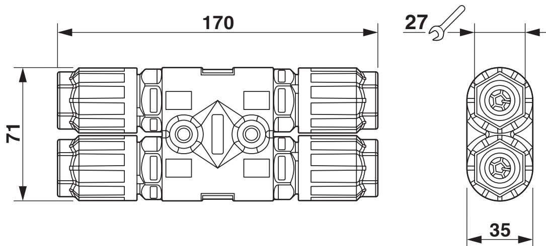
Rysunek wymiarowy
