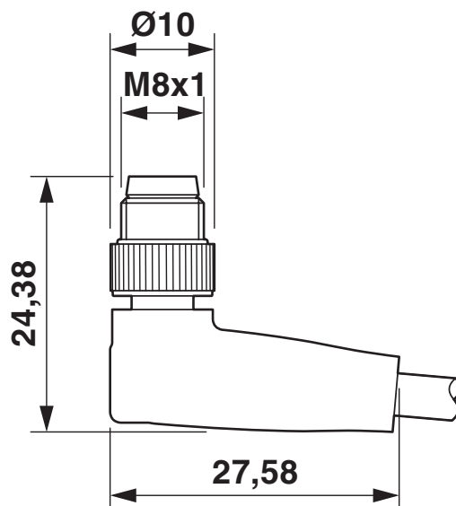
Rysunek wymiarowy
