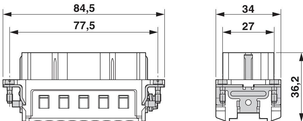
Rysunek wymiarowy
