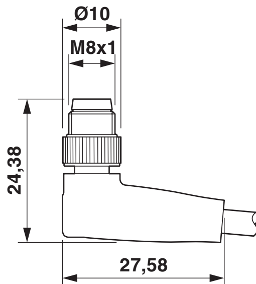
Rysunek wymiarowy
