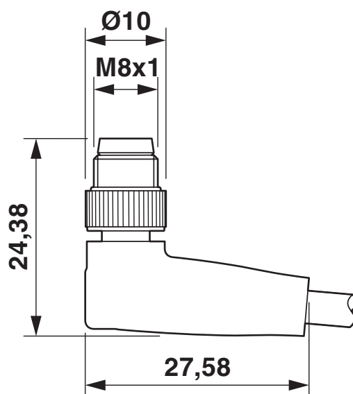
Rysunek wymiarowy
