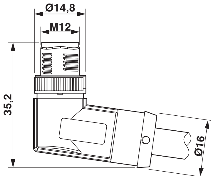
Rysunek wymiarowy
