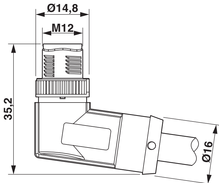
Rysunek wymiarowy
