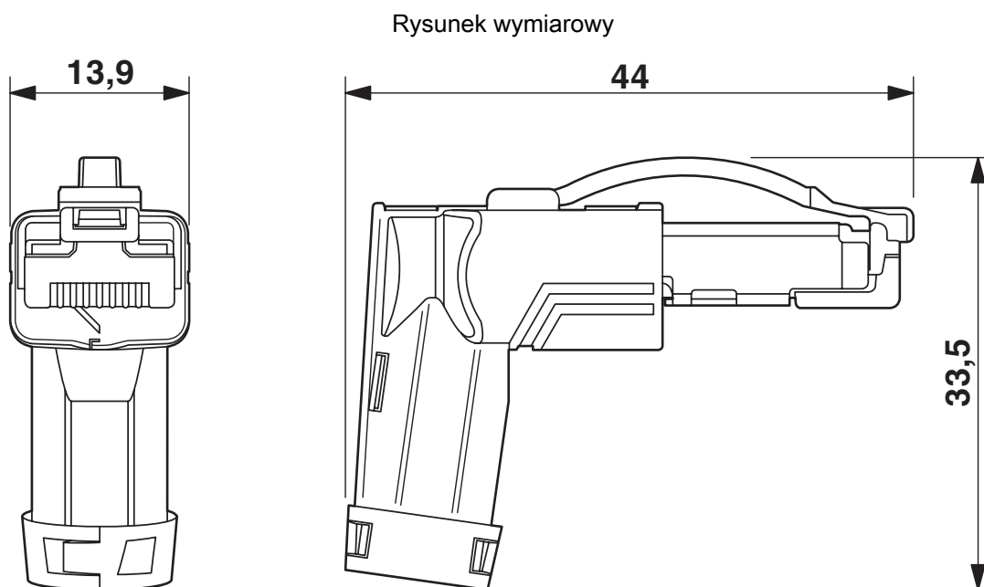
złącze wtykowe RJ45, IP20, kątowne
