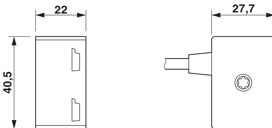
Rysunek wymiarowy
