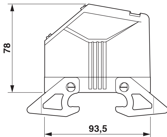
Rysunek wymiarowy
