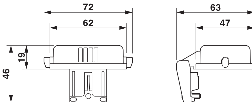
Rysunek wymiarowy
