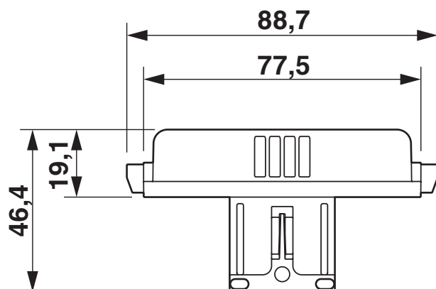
Rysunek wymiarowy
