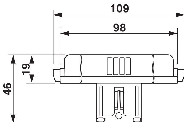
Rysunek wymiarowy
