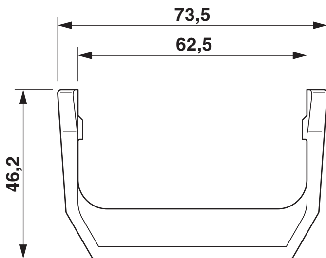
Rysunek wymiarowy
