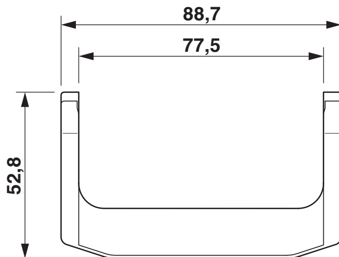
Rysunek wymiarowy
