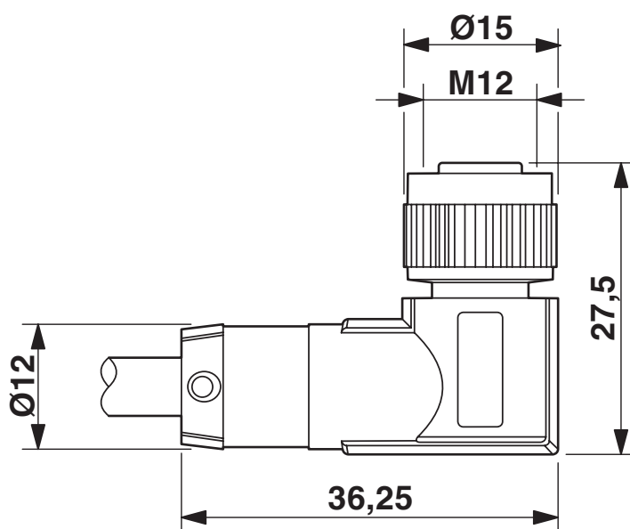
Rysunek wymiarowy
