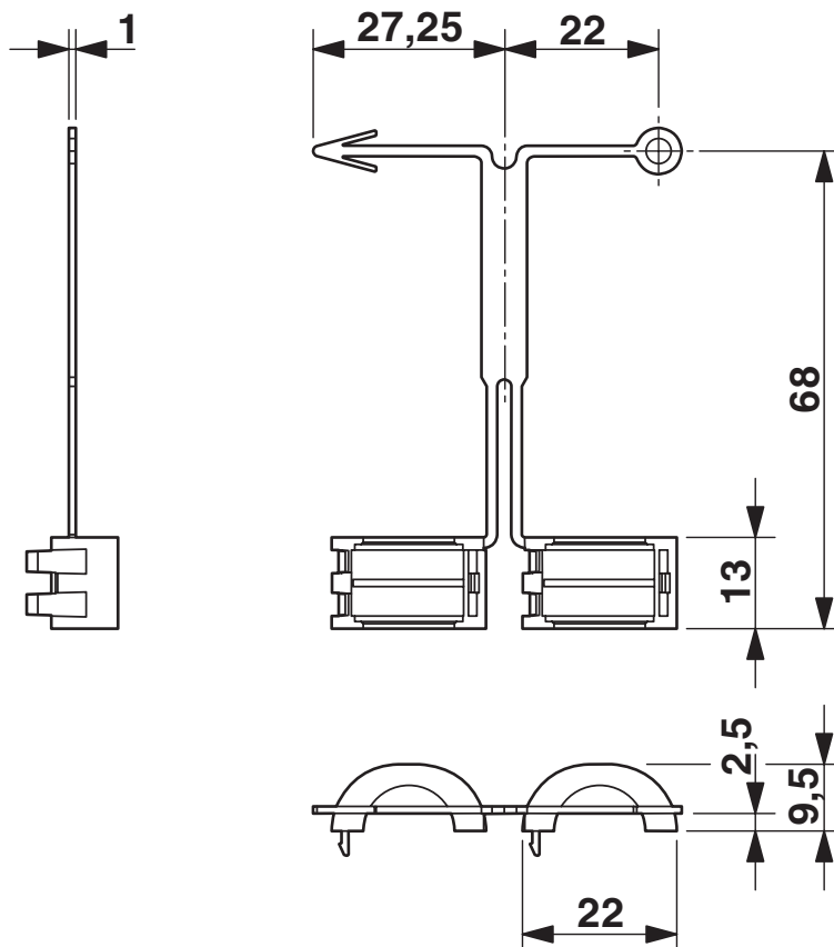
Rysunek wymiarowy
