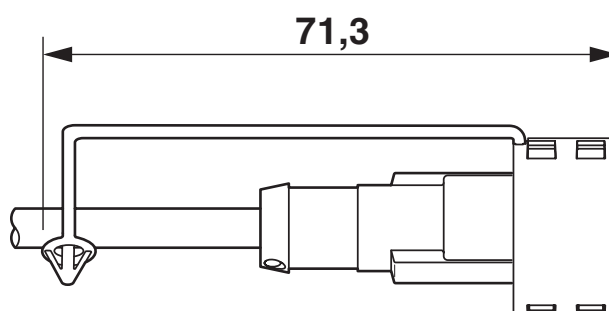
Rysunek wymiarowy
