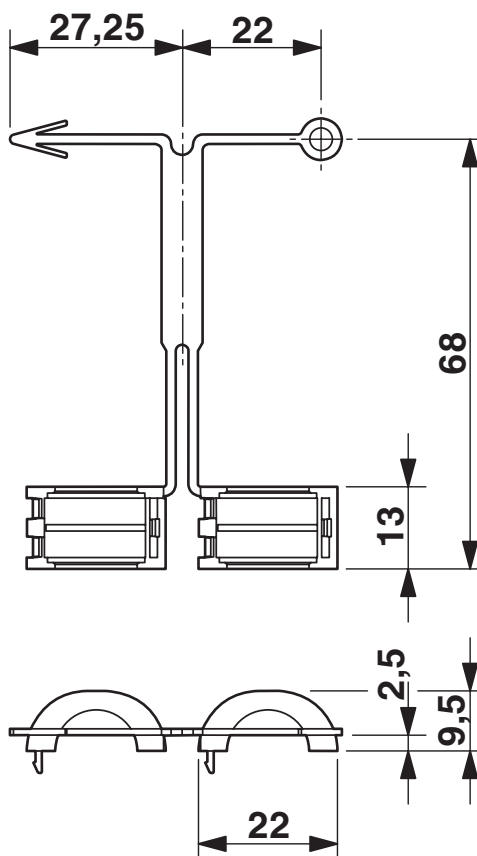
Rysunek wymiarowy
