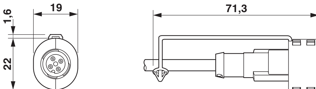
Rysunek wymiarowy
