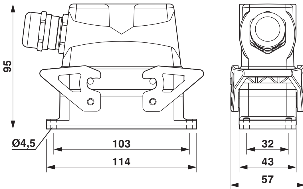
Rysunek wymiarowy
