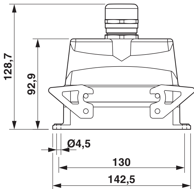
Rysunek wymiarowy
